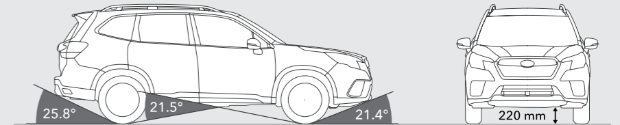
أدنى خلوص للطريق Minimum Road Clearance زاوية الاقتراب Approach Angle زاوية التخطي Break-over Angle زاوية الإقلاع Departure Angle
